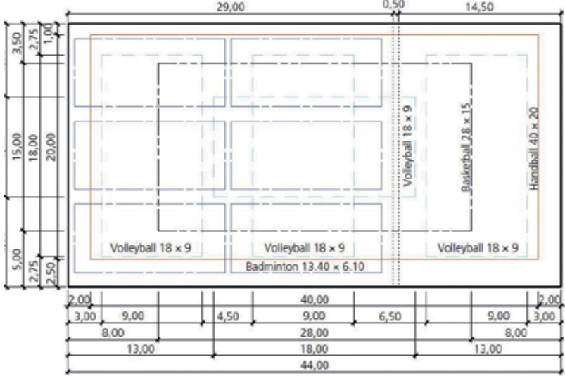
Die Dimensionen einer Doppeltturnhalle des Typs B.
